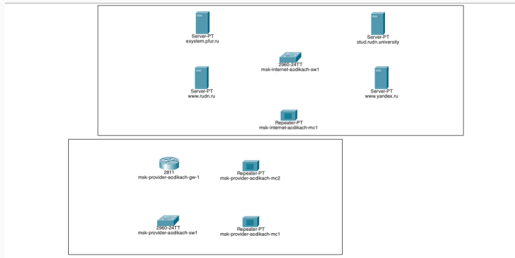
Рис. 5: Размещение
