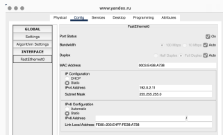
Рис. 11: Настройка www.yandex.ru
