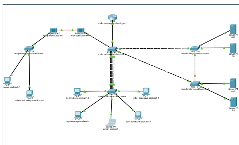
Рис. 2.1: Изменённая топология
