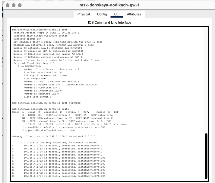
Рис. 2: Проверка состояния протокола OSPF на маршрутизаторе
