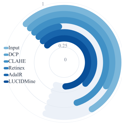
SSIM ↑
