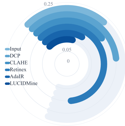
MAE ↓
