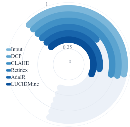
Vis ↑
