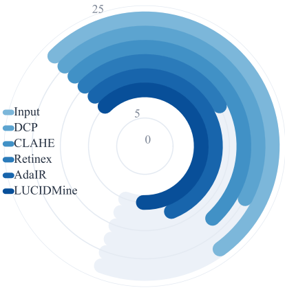
PSNR ↑
