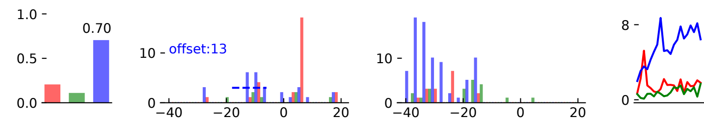
Frame distr.
