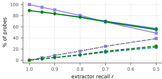
budget 2k
