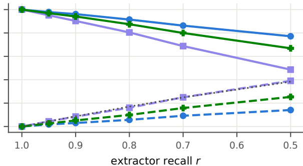
budget 8k
