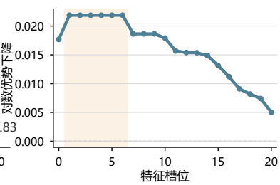
局部遮挡曲线
