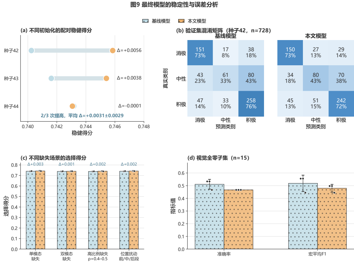
图 9 最终模型的稳定性与误差分析。(a) 三个训练种子下与对应基线的配对鲁棒分数；(b) 种子 42 的干净验证集混淆矩阵，行为真实类别、列为预测类别；(c) 按缺失形式汇总的选择分数；(d) 15 条视觉整段原生全零样本的分类准确率与宏平均 F1。误差线表示三次训练种子的样本标准差，不表示置信区间。
