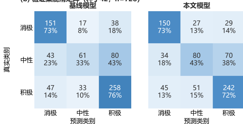
(b) 验证集混淆矩阵 (种子42, n=728)
