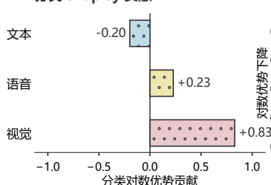
分类 Shapley 贡献
