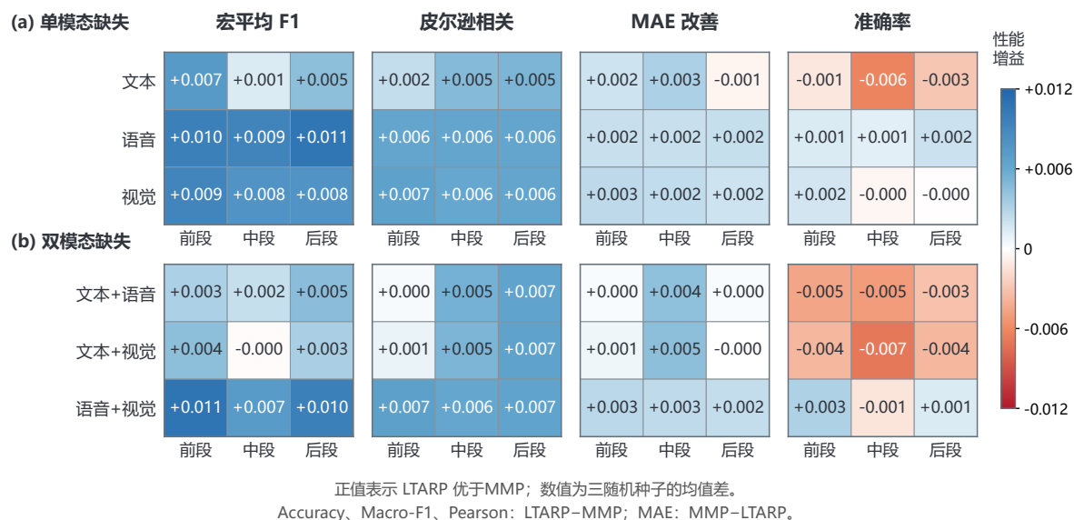
图 12 最终鲁棒配置与 MMP 基线在不同缺失场景下的指标差异。MAE 取 MMP 减 LTARP，其余指标取 LTARP 减 MMP；正值表示 LTARP 对应指标更优。
