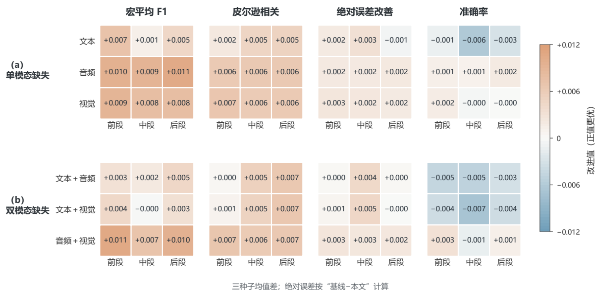
图 6 缺失模态及位置对模型间性能差异的影响。宏平均 F1、相关系数和准确率为“本文模型减基线模型”，MAE 为“基线模型减本文模型”，故正值均表示本文模型较优；色块为验证集三次随机初始化均值之差。
