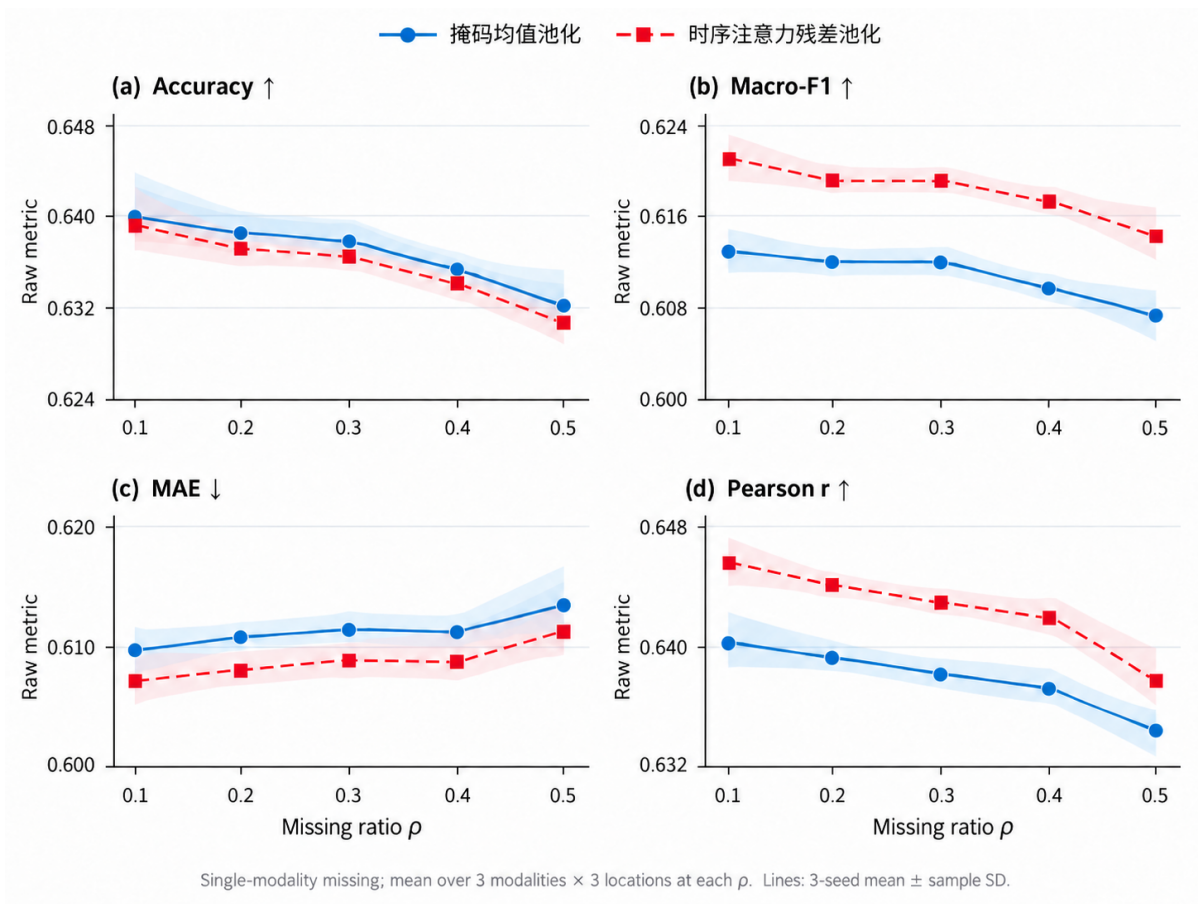
图 5 不同单模态连续缺失比例下的验证集性能。每个比例先对三种模态与前、中、后三种遮挡位置取平均，再绘制三次随机初始化的均值与样本标准差；阴影为样本标准差。蓝线为掩码均值池化基线，红线为时间注意力残差池化模型；MAE 越低越好，其余指标越高越好。
