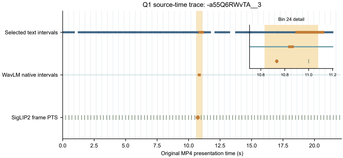
图 3 典型样本的三模态时间映射与来源追踪。阴影表示第 24 个统一时间窗，局部图放大其源时间位置。
