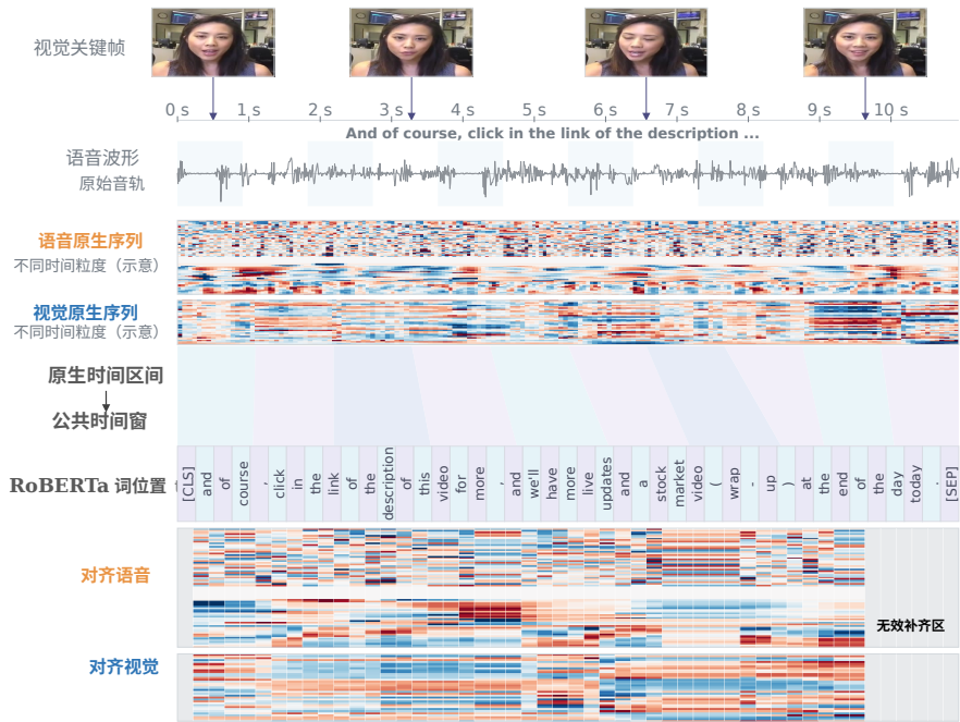
图 2 三模态原生时间轴到公共时间窗的映射示意。文本片段、音频帧和视觉采样帧首先关联各自的媒体时间；统一时间窗根据正时间交叠选择原生特征，并记录有效位与来源。图中热图及采样间隔只用于展示时间粒度差异，不代表本文实际特征值或采样率。
