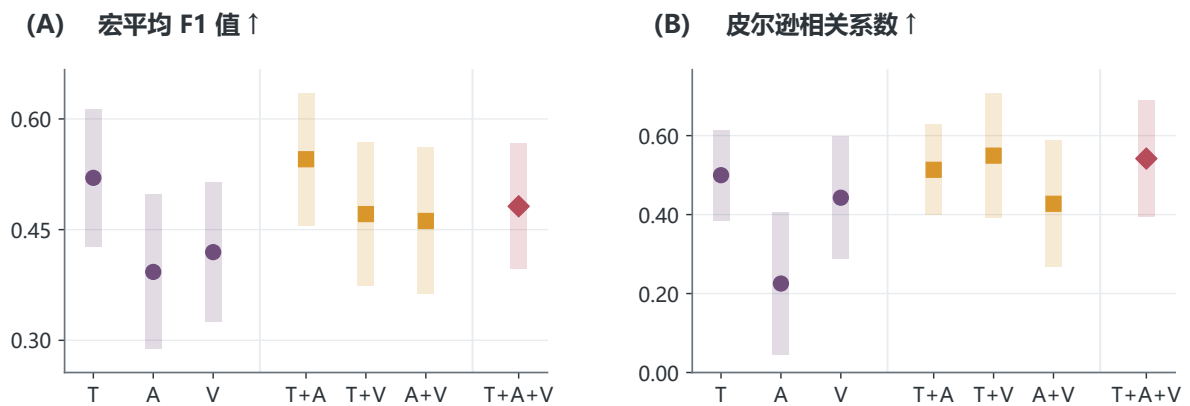
图 A2 不同模态组合的辅助评价结果。点表示均值，独立的半透明区间表示均值上下一个标准差；圆形、方形和菱形分别表示单模态、双模态和三模态组合。
