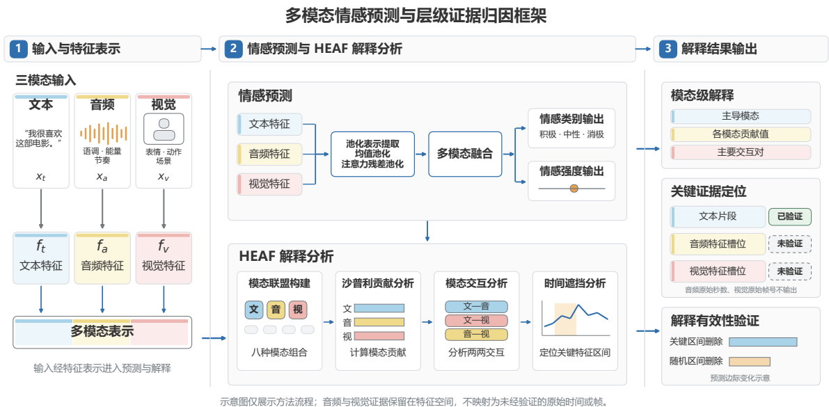
图 8 多模态情感预测与层级证据归因框架。三模态联盟用于模态贡献和交互分析，连续遮挡定位特征空间关键区间；原始文本证据可核验，音频与视觉的秒数和帧号映射尚未核
