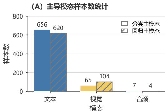
图8 基于验证集的解释有效性与主导模态统计
