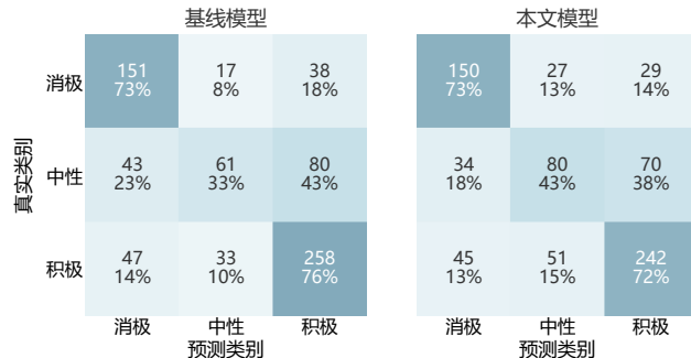
(b) 验证集混淆矩阵 (种子42, n=728)
