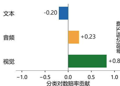
模态 Shapley 贡献
