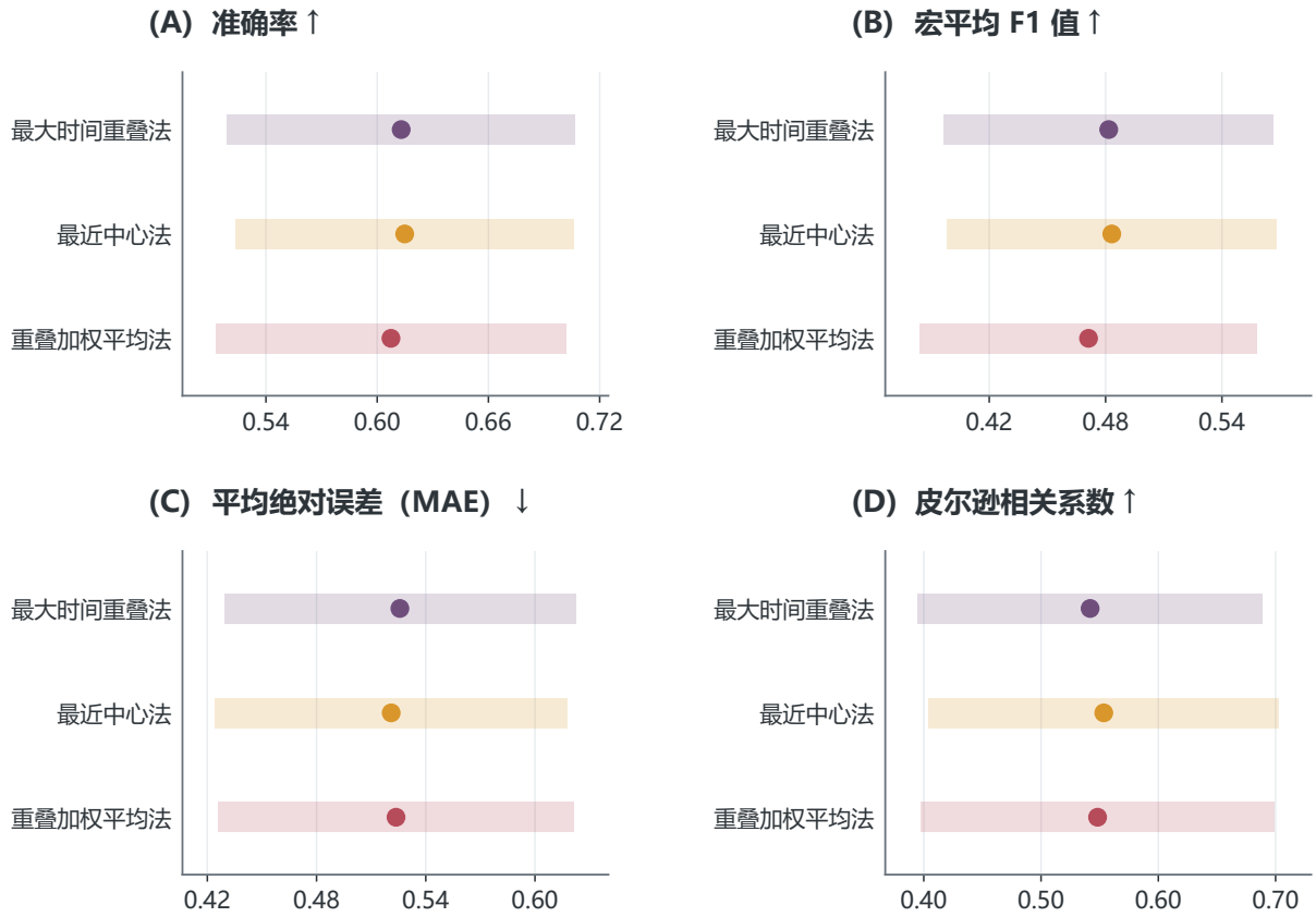
图 7 不同时序对齐方法的辅助评价结果。点表示重复分层五折评价均值，半透明区间表示均值上下一个样本标准差。该评价仅用于比较不同特征构建方案的信息保持情况，不作为独立泛化性能或统计显著性结论。
