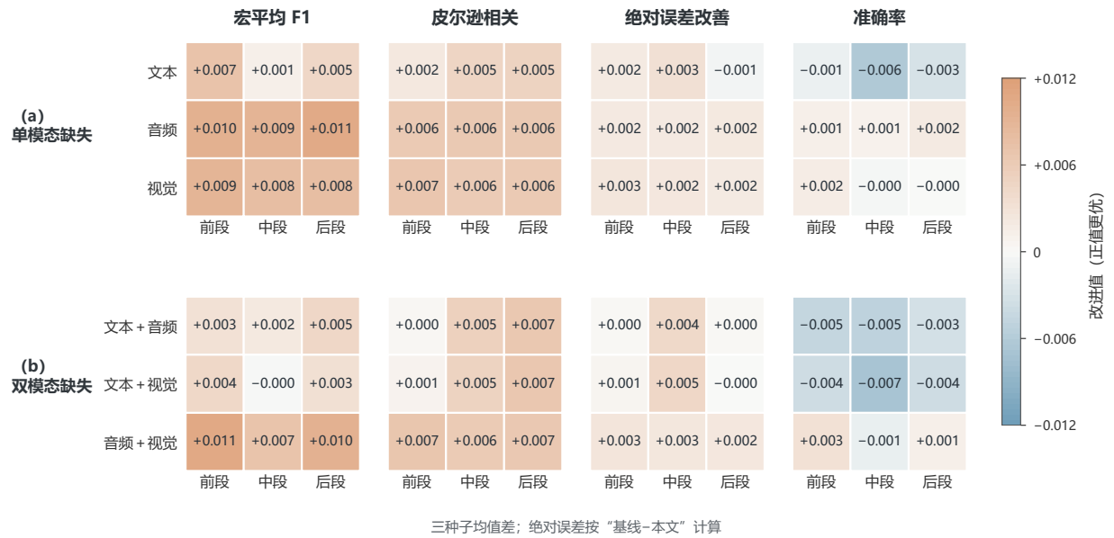
图 12 缺失模态及位置对模型间性能差异的影响。宏平均 F1、相关系数和准确率为“本文模型减基线模型”，MAE 为“基线模型减本文模型”，故正值均表示本文模型较优；色块为验证集三次随机初始化均值之差。
