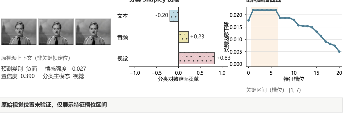
图 16 附件 4 两条典型样本的层级解释。样本 14 给出已核验文本片段；样本 02 只定位视觉特征槽位，视频帧为原视频上下文展示，不表示算法定位出的关键帧。
