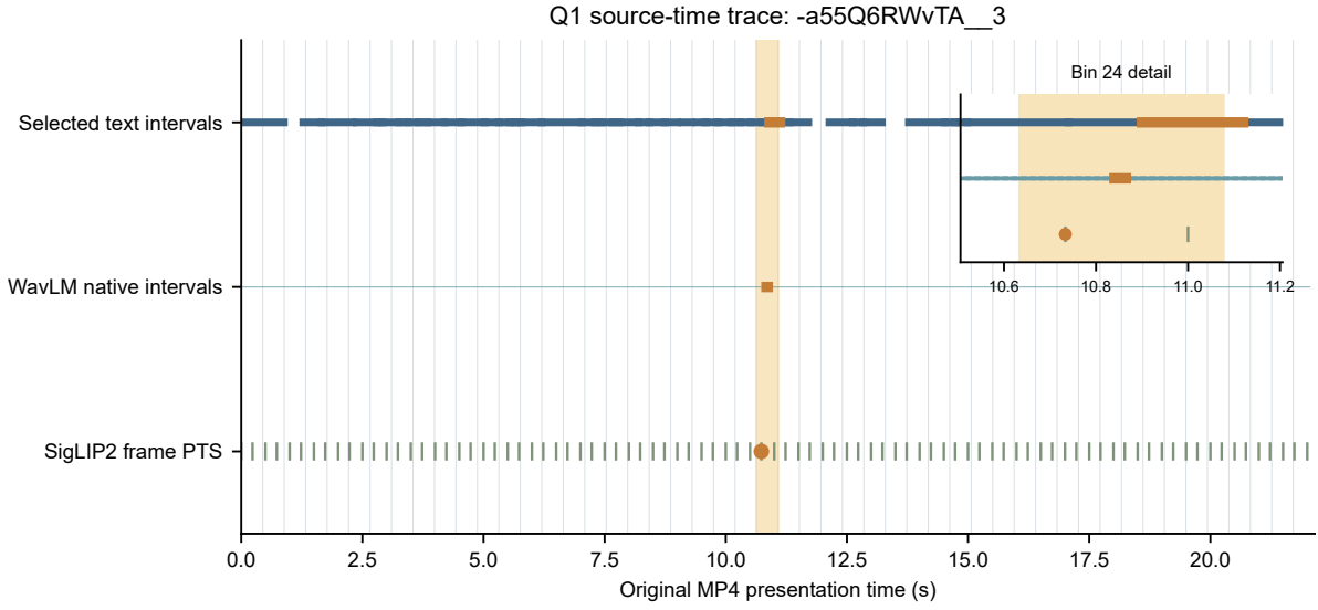
图 8 典型样本的三模态时间映射与来源追踪。以样本 -a55Q6RWvTA__3 为例，展示视觉采样帧显示时间、语音原生特征时间区间和文本特征区间，并放大第 24 个公共时间窗对应的原生来源。该图用于验证统一时间位置能够回溯至实际媒体时间。
