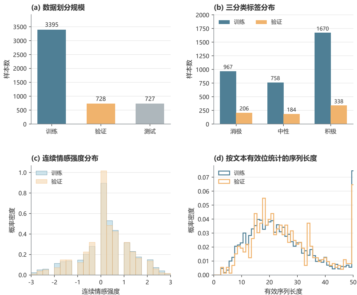
图 10 附件 2 aligned-50 特征的数据划分与标签统计。(a) 训练、验证和测试划分的样本规模；(b) 训练集与验证集的三分类标签分布；(c) 连续情感强度分布；(d) 根据文本有效位字统计的有效序列长度分布。测试划分仅展示样本数量，不参与标签统计、模型选择或性能分析。
