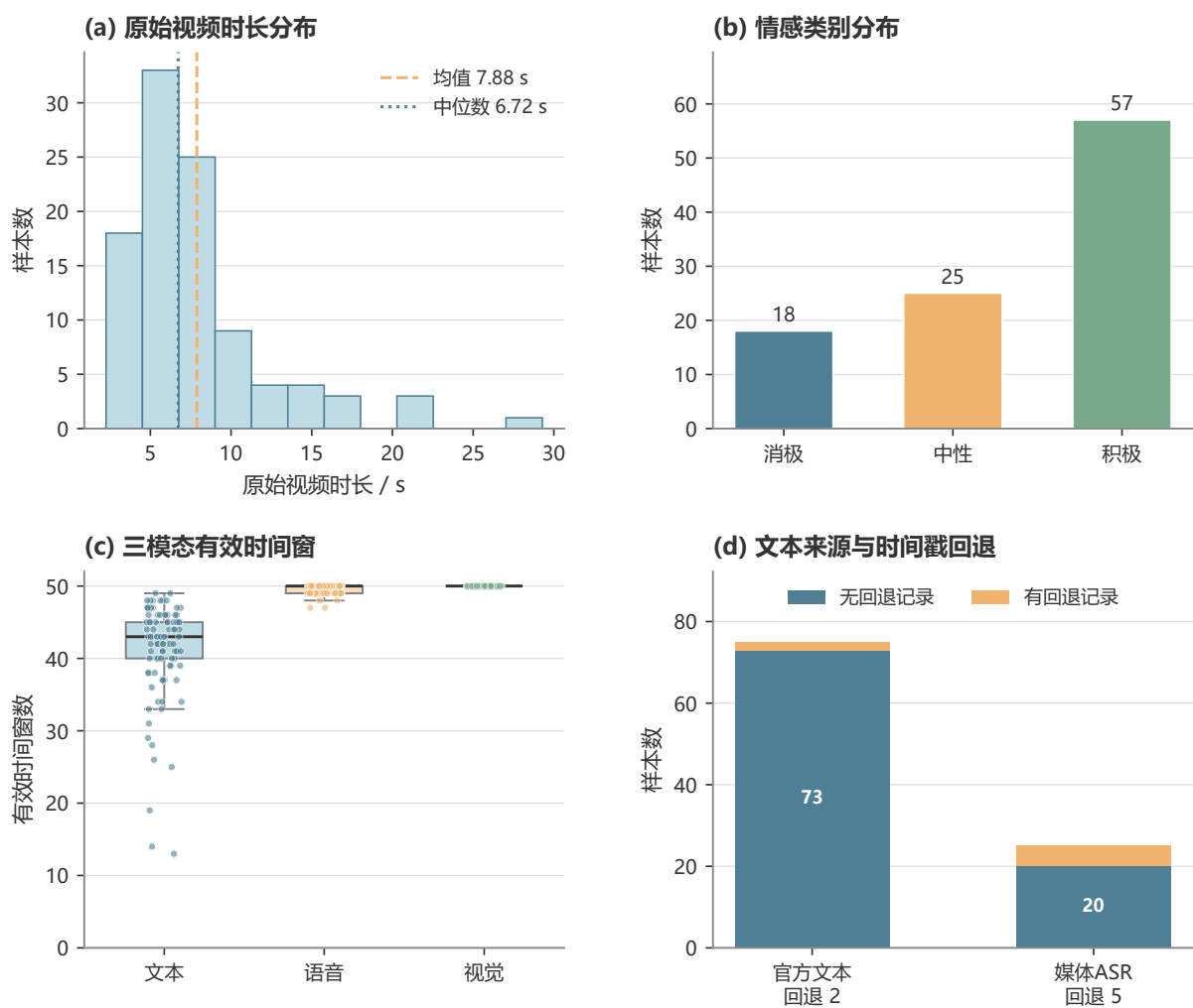
图 5 附件 1 原始样本及特征覆盖的描述性统计。(a) 100 条视频的原始时长分布；(b) 三类情感标签样本数量；(c) 文本、语音和视觉在 50 个公共时间窗中的有效位置分布；(d) 文本来源及时间戳回退情况。统计均由最终 Q1 处理清单直接计算。
