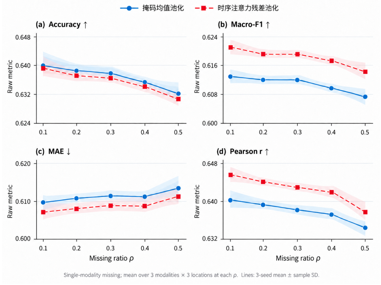
图 11 不同单模态连续缺失比例下的验证集性能。每个比例先对三种模态与前、中、后三种遮挡位置取平均，再绘制三次随机初始化的均值与样本标准差；阴影为样本标准差。蓝线为掩码均值池化基线，红线为时间注意力残差池化模型；MAE 越低越好，其余指标越高越好。
