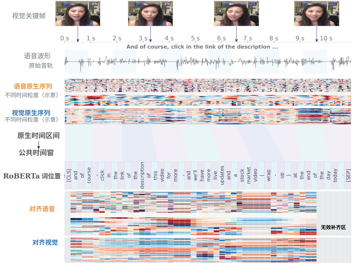
图 6 三模态原生时间轴到公共时间窗的映射示意。文本片段、音频帧和视觉采样帧首先关联各自的媒体时间；统一时间窗根据正时间交叠选择原生特征，并记录有效位与来源。
