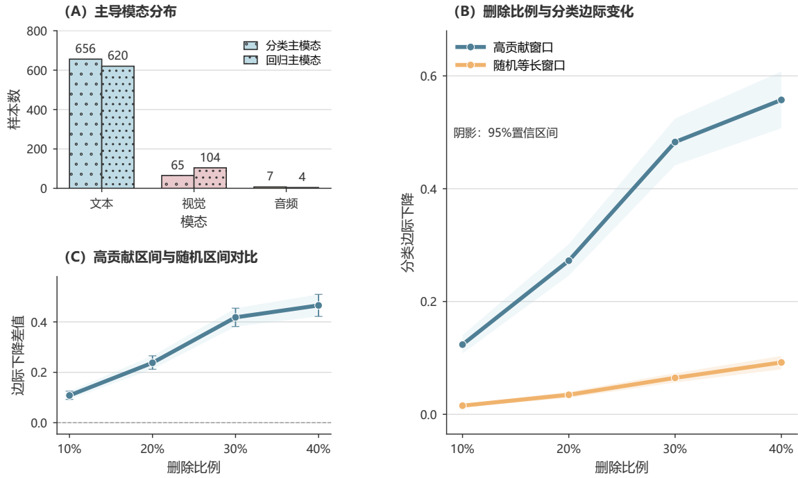
图 15 验证集上的主导模态与删除干预结果。(A) 728 条样本的分类/回归主导模态计数；(B) 审计子集上所选与随机窗口的分类边际下降及视频分组 95% 区间；(C) 两种删除方式的配对差。所选窗口来自同一候选集合的最大影响值，因此相对随机窗口的优势含选择效应。
