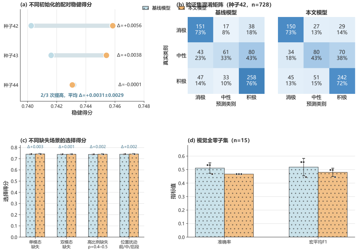
图 13 最终模型的稳定性与误差分析。(a) 三个训练种子下与对应基线的配对鲁棒分数；(b) 种子 42 的干净验证集混淆矩阵，行为真实类别、列为预测类别；(c) 按缺失形式汇总的选择分数；(d) 15 条视觉整段原生全零样本的分类准确率与宏平均 F1。误差线表示三次训练种子的样本标准差，不表示置信区间。
