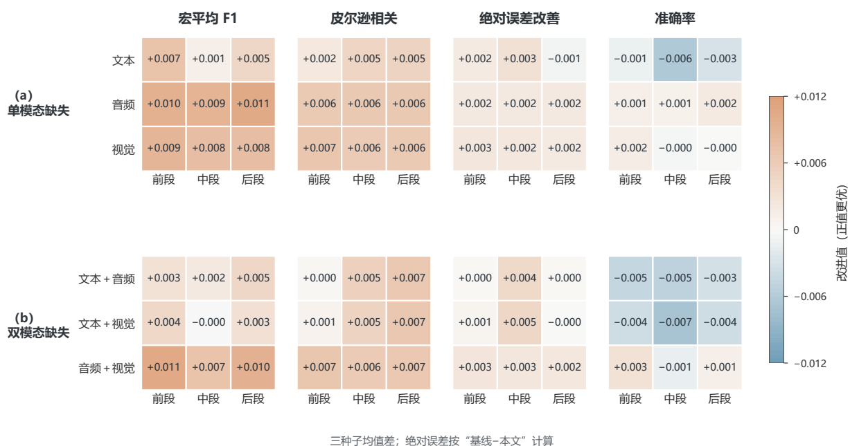
图 12 缺失模态及位置对模型间性能差异的影响。宏平均 F1、相关系数和准确率为“本文模型减基线模型”，MAE 为“基线模型减本文模型”，故正值均表示本文模型较优；色块为验证集三次随机初始化均值之差。
