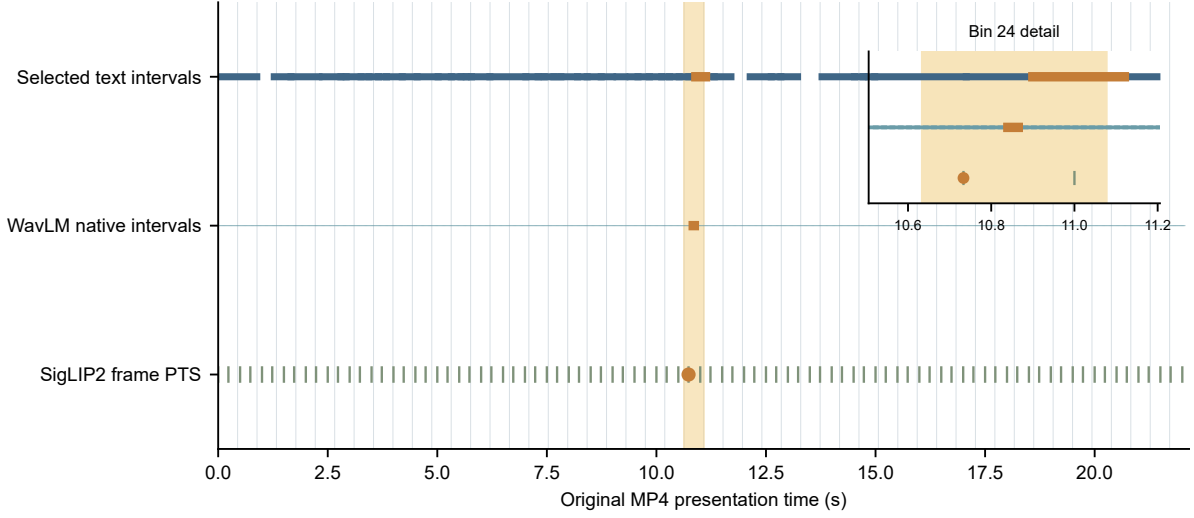
图 8 典型样本的三模态时间映射与来源追踪。以样本 -a55Q6RWvTA__3 为例，展示视觉采样帧显示时间、语音原生特征时间区间和文本特征区间，并放大第 24 个公共时间窗对应的原生来源。该图用于验证统一时间位置能够回溯至实际媒体时间。
