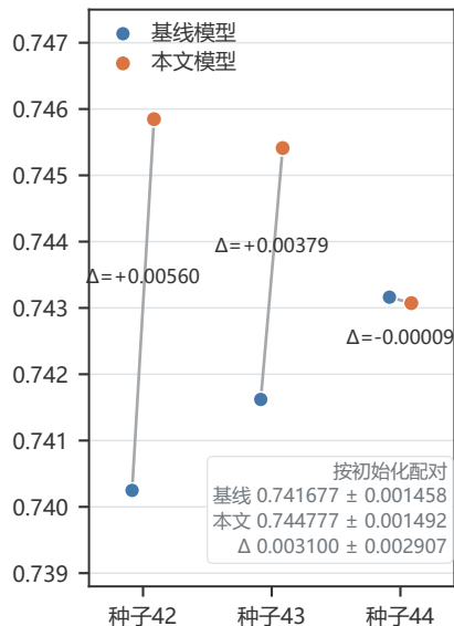
(A) 鲁棒分数 (按初始化配对)
