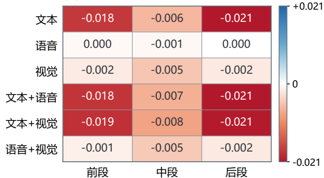
(b) 宏平均 F1 变化
