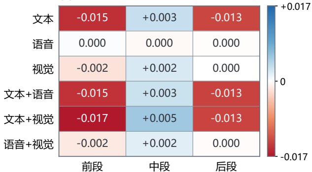
(c) MAE 变化
