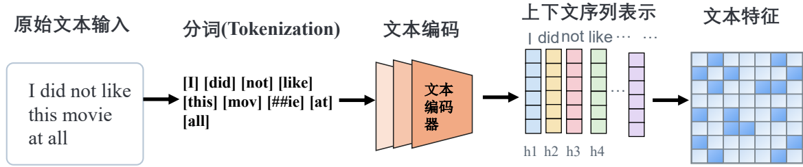
图 4 文本模态特征提取流程。色块为表示结构示意图。
