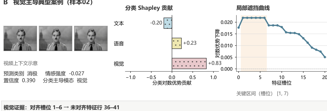
图 18 附件 4 的典型样本。（A）样本 14 的文本贡献、局部遮挡曲线与原文片段；（B）样本 02 的视觉贡献、局部遮挡曲线与未对齐特征行对应。浅色带标出所选特征区间，视频画面为上下文示意。
