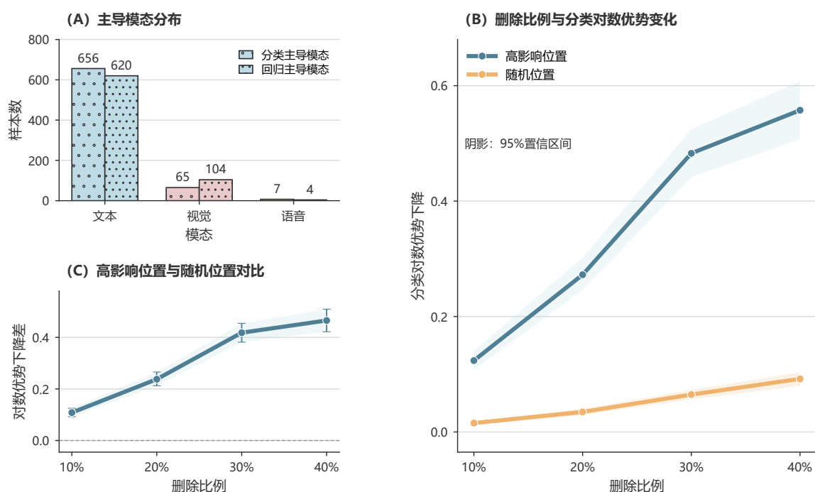
图 17 主导模式与删除干预结果。(A) 728 条验证样本的分类、回归主导模式计数；(B) 396 条独立验证样本的删除比例曲线；(C) 高影响位置与随机位置的配对下降差。阴影为按视频分组的 95% 自助采样区间。
