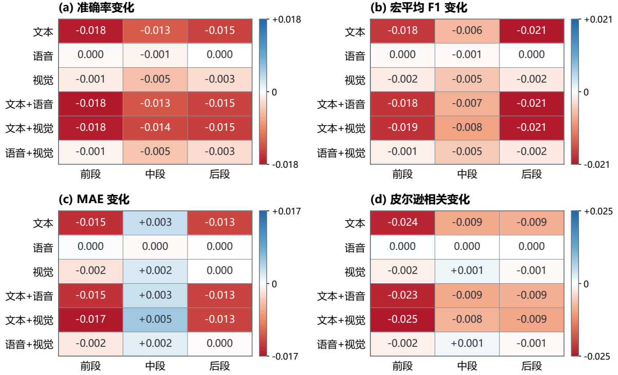
图 12 不同模态与缺失位置相对完整输入的指标变化（目标缺失比例 \rho_{\text{target}} = 0.3 ）。数值为三次随机初始化的配对均值，各指标使用独立色标；MAE 采用“完整输入 - 缺失输入”，其余指标采用“缺失输入 - 完整输入”，因此正值均表示性能改善。
