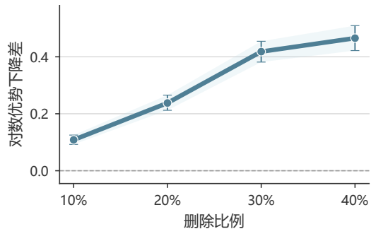
(C) 高影响位置与随机位置对比
