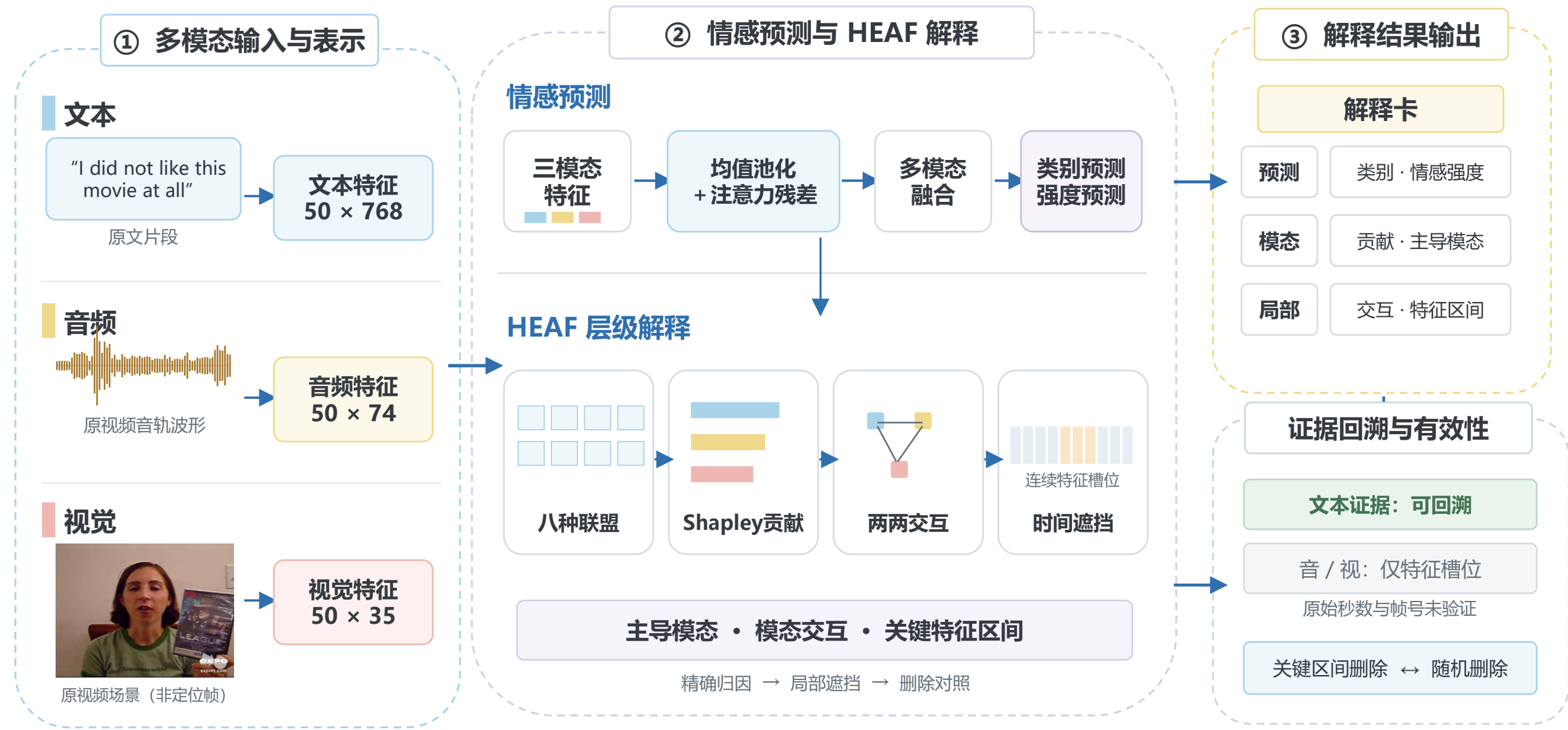
图7 多模态情感预测与层级证据归因框架
