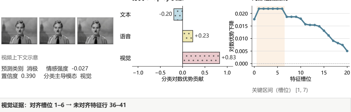
图 18 附件 4 的典型样本。（A）样本 14 的文本贡献、局部遮挡曲线与原文片段；（B）样本 02 的视觉贡献、局部遮挡曲线与未对齐特征行对应。浅色带标出所选特征区间，视频画面为上下文示意。
