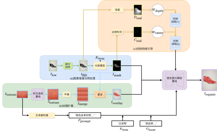
图 3-1 算法概述
