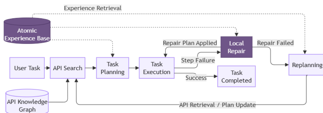
圖 3.1: CBR-APIKGAgent 系統架構圖
