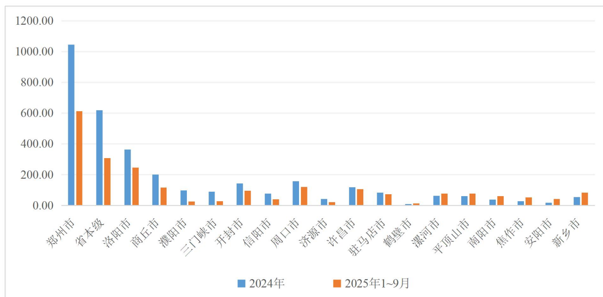
图 3.4 河南省省本级及各地市城投企业债券发行情况（单位：亿元）
