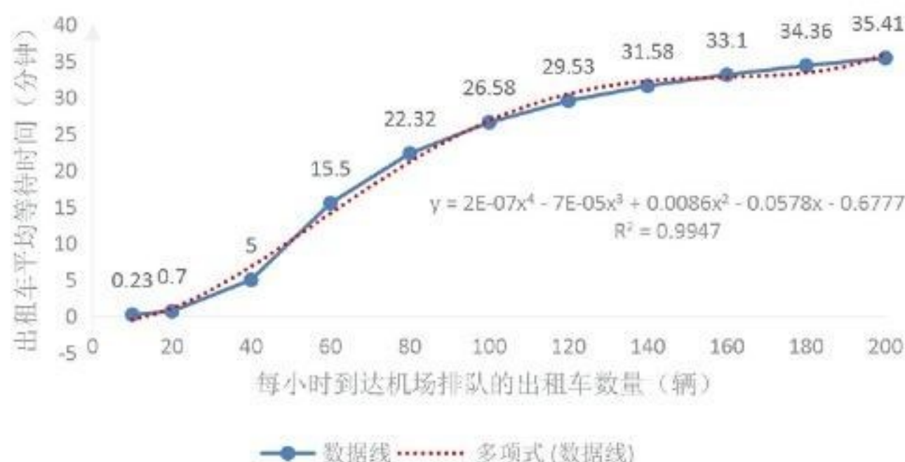
图5-12 1.5小时模拟的数据曲线及拟合曲线
