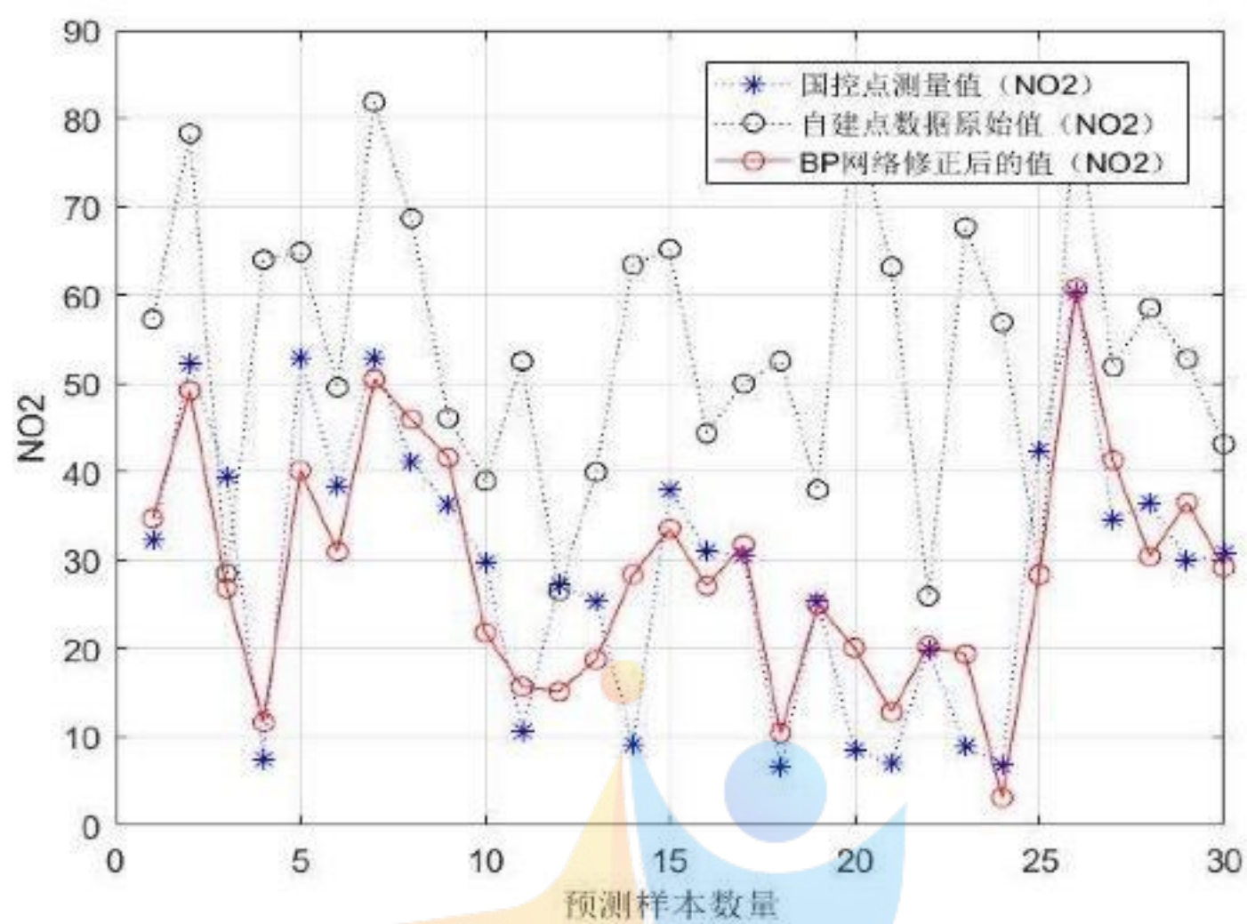
图 21 NO 2 预测效果对比图
