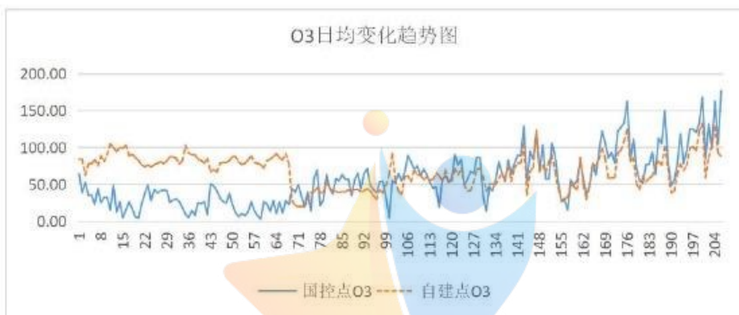
图 11 O 3 日均变化趋势图
