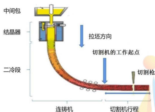
图 1 连铸工艺的示意图
