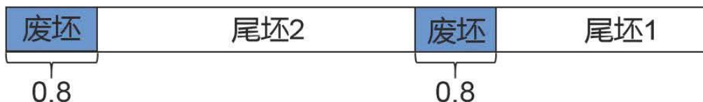
图 5 “尾坯 1+0.8 米废坯+尾坯 2+0.8 米废坯”的情况
