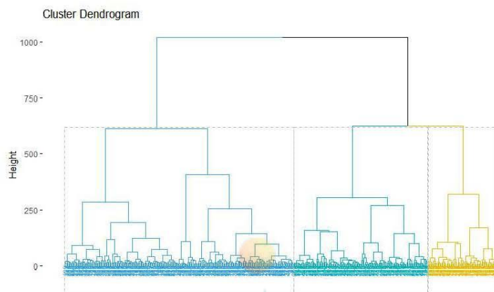
图 4-20. Ward 聚类谱系图
