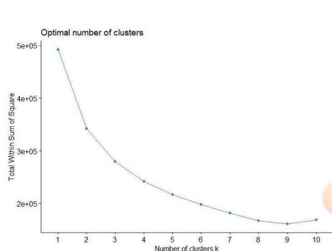
图 4-12.肘部法则确定聚类数
