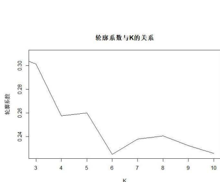
图 4-18.平均轮廓法确定聚类数
