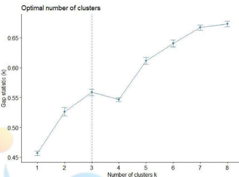
图 4-13.间隔统计量确定聚类数
