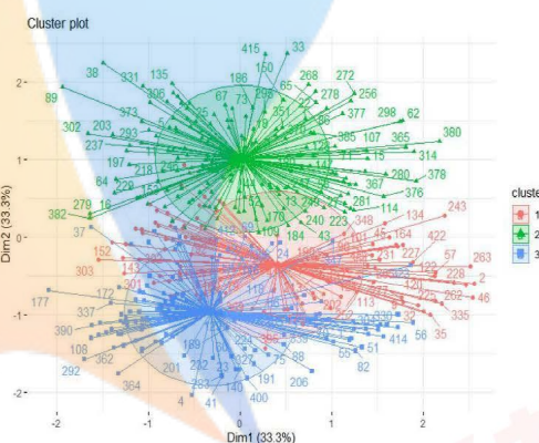
图 4-11.K-means 聚类结果图
