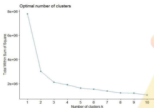
图 4-8.肘部法则确定聚类数
