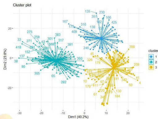
图 4-19.K-means 聚类结果图
