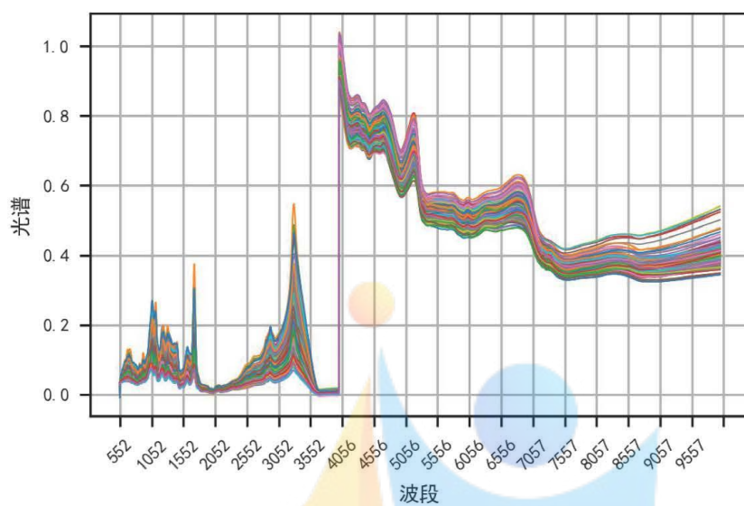
图8 附件3 中红外近红外合并数据
