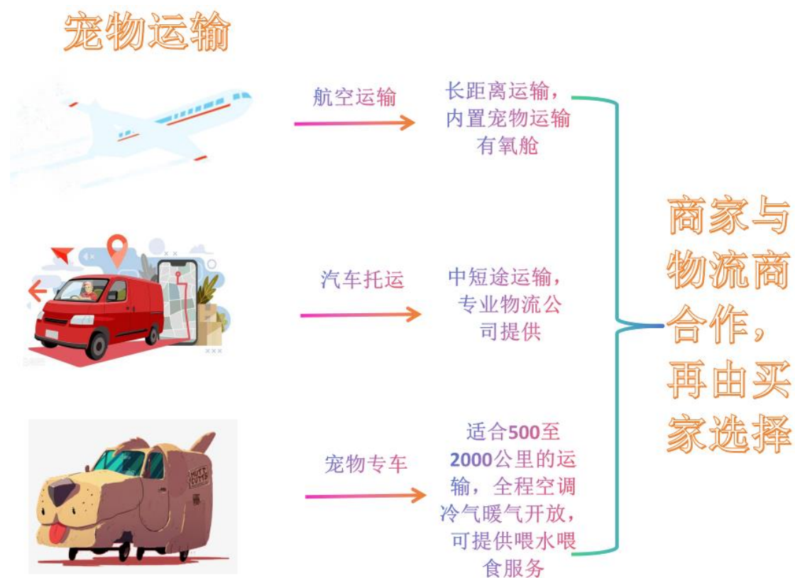
图 6-4 物流模式图
