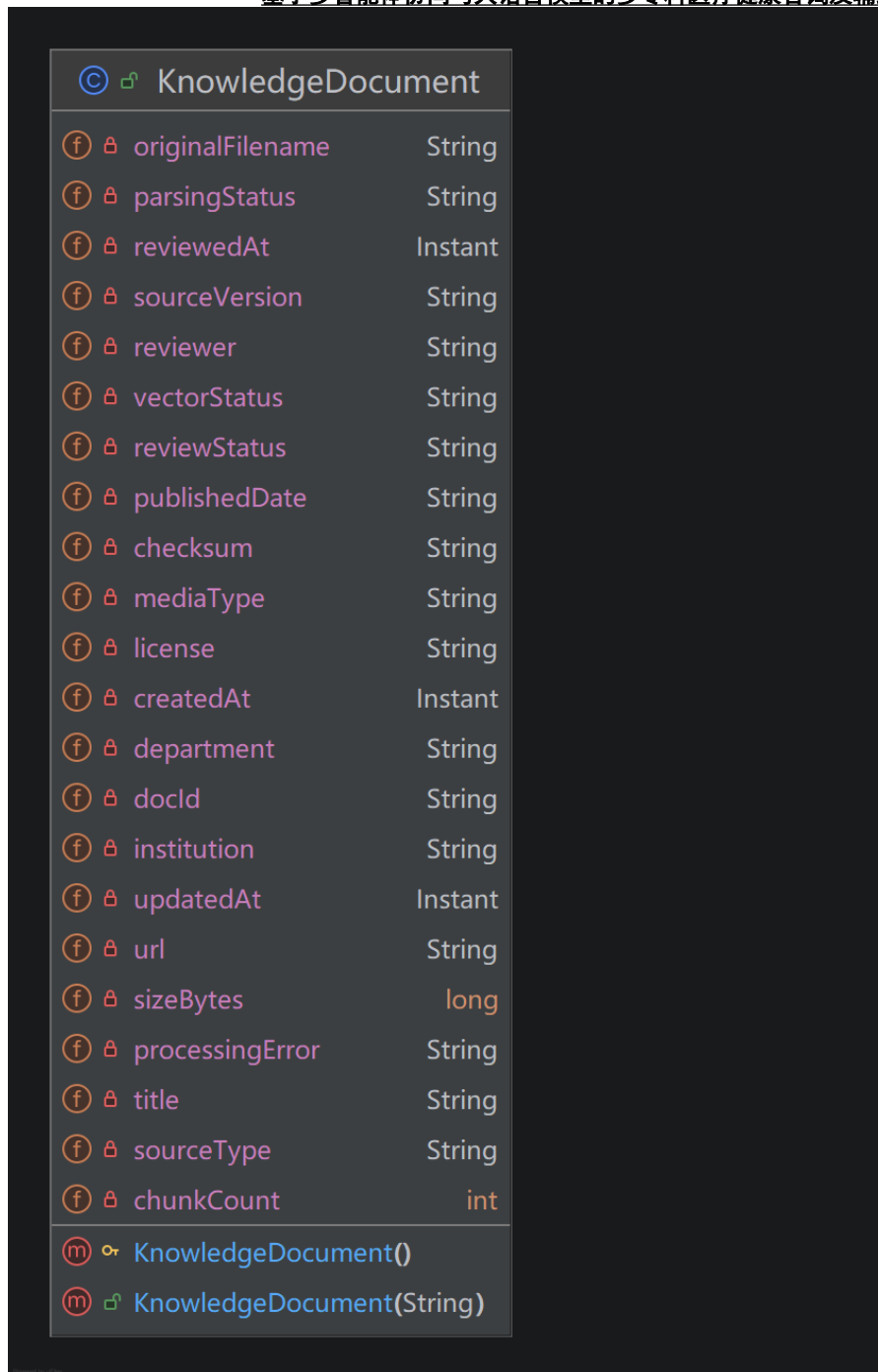
图 3-15 KnowledgeDocument 实体类图
