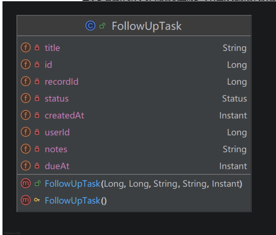
图 3-14 FollowUpTask 实体类图
