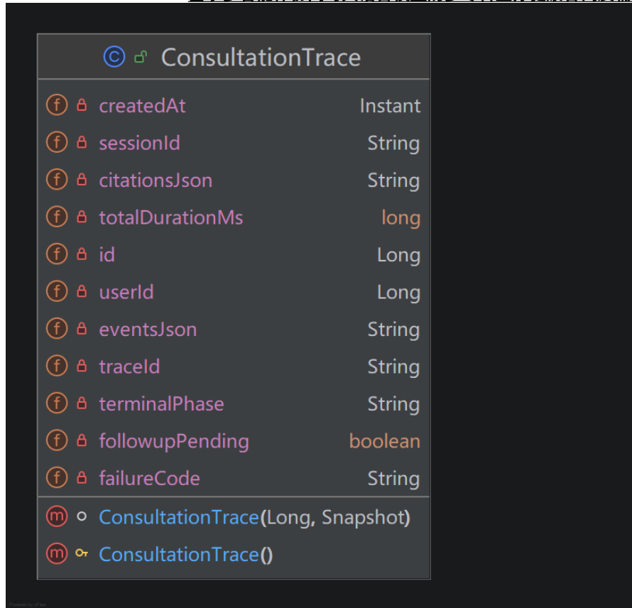
图 3-12 ConsultationTrace 实体类图
