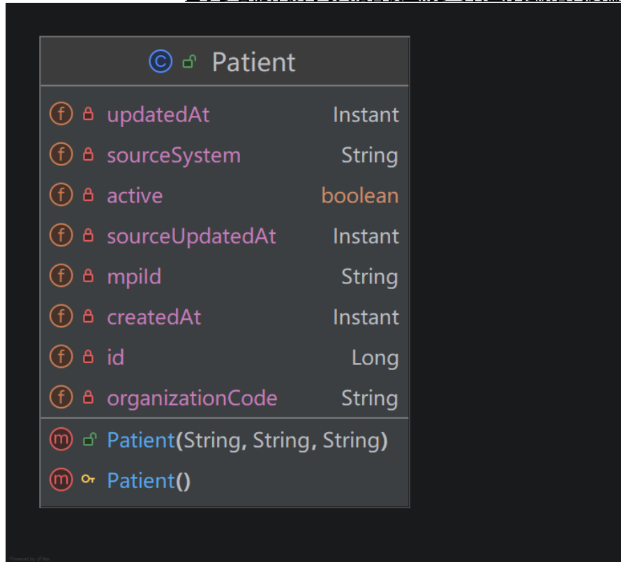
图 3-8 Patient 实体类图
