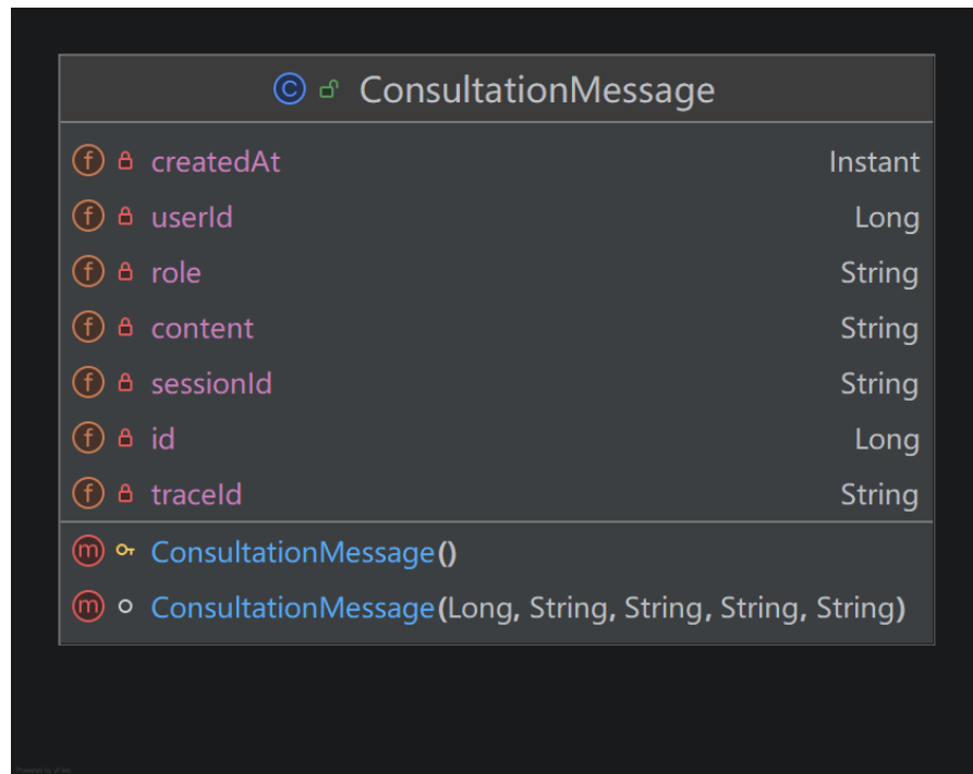
图 3-11 ConsultationMessage 实体类图
