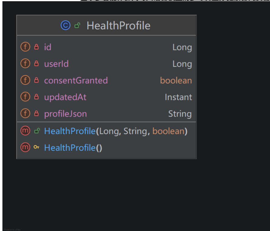
图 3-13 HealthProfile 实体类图
