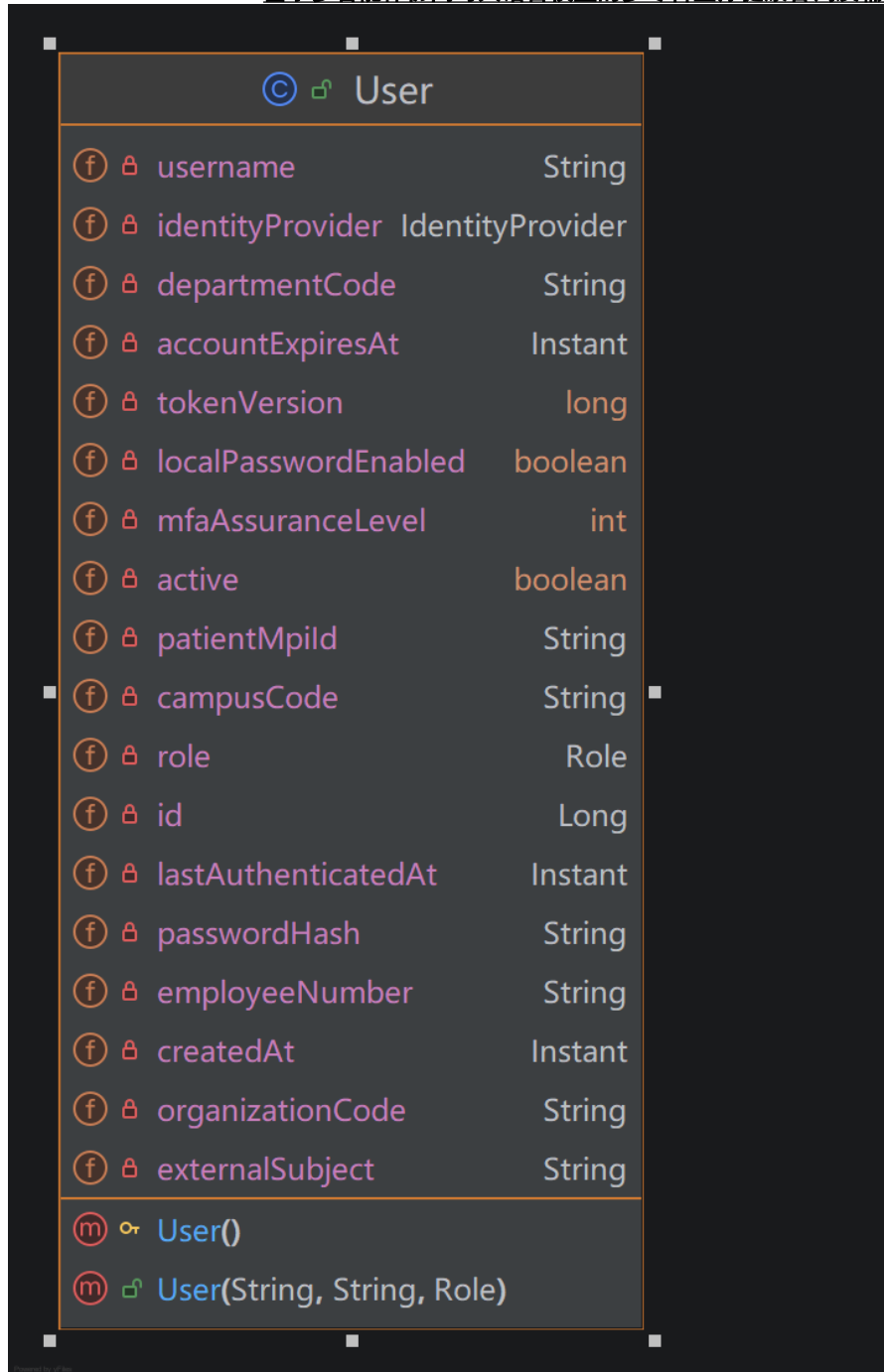
图 3-7 User 实体类图
