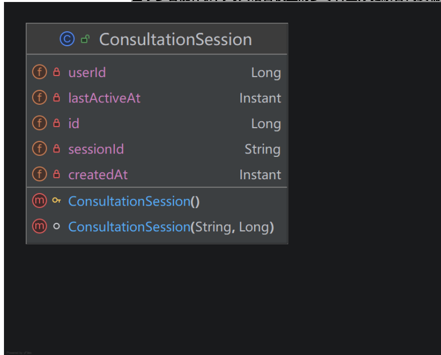
图 3-9 ConsultationSession 实体类图
