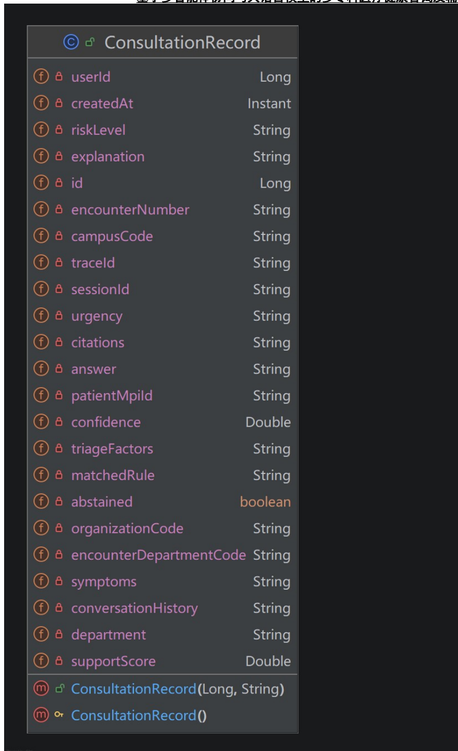
图 3-10 ConsultationRecord 实体类图
