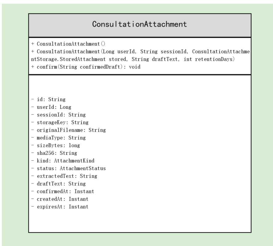
图 3-13 ConsultationAttachment 实体类图
