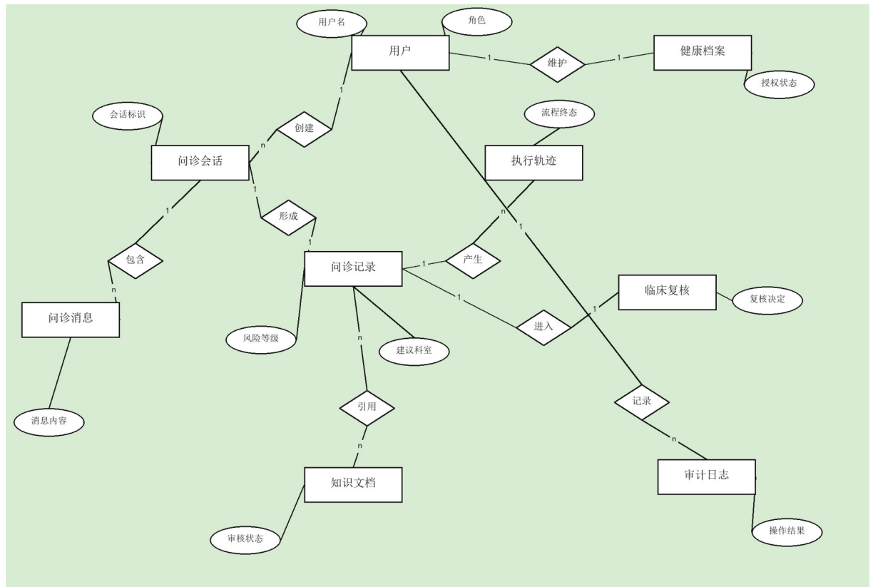
图 3-4 E-R 图
