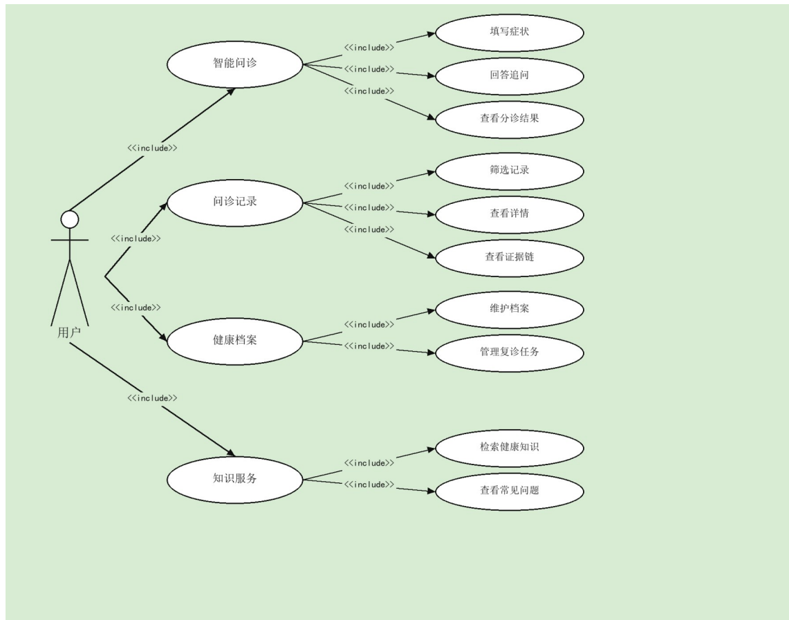
图 3-5 用户用例图
