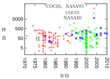
图1 本研究中学习者使用的项目。图4展示了项目属性。COC81是1981年COCOMO书籍(Boehm, 1981年)中的原始数据。这些数据来自1970年至1980年的项目。NASA93是美国国家航空航天局(NASA)在20世纪90年代初收集的关于支持国际空间站规划活动的软件的数据。我们的其他数据集是NASA10和COC05(后者属于专有数据,无法向研究界发布)。非专有数据(COC81、NASA93和NASA10)可在 http://openscience.us/repo 获取,或见图3。
