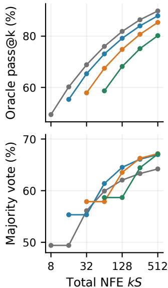
GSM8K Pre-NFT
