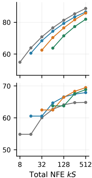
GSM8K Post-NFT
