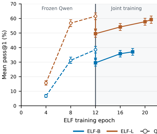
GSM8K
