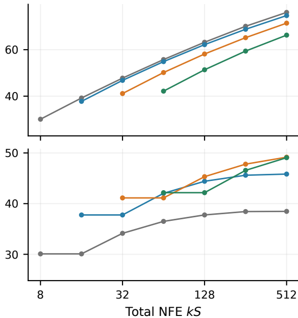
GSM8K LFRM-B · post-NFT
