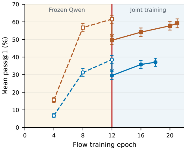
GSM8K
