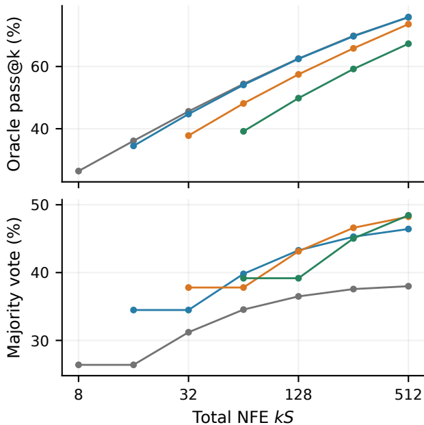
GSM8K CEDR-B · pre-NFT
