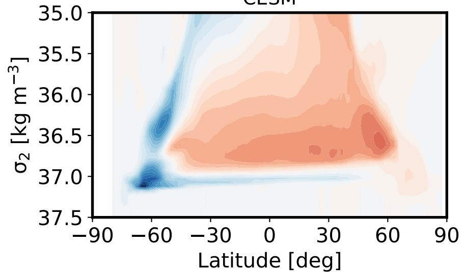
CESM
