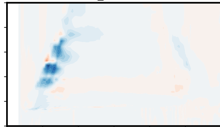
GFDL_BV - GFDL
