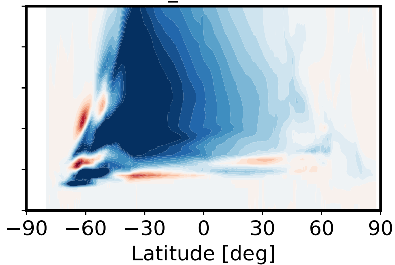
CESM_MBK - CESM
