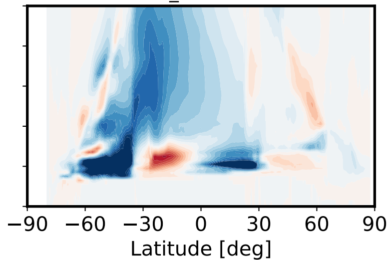
CESM_LBK - CESM
