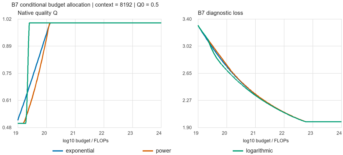
图 5.6 B7 条件模型在 8192 Token 下的质量选择及 Loss 随预算变化。曲线平台受矩形支持域上界约束。
