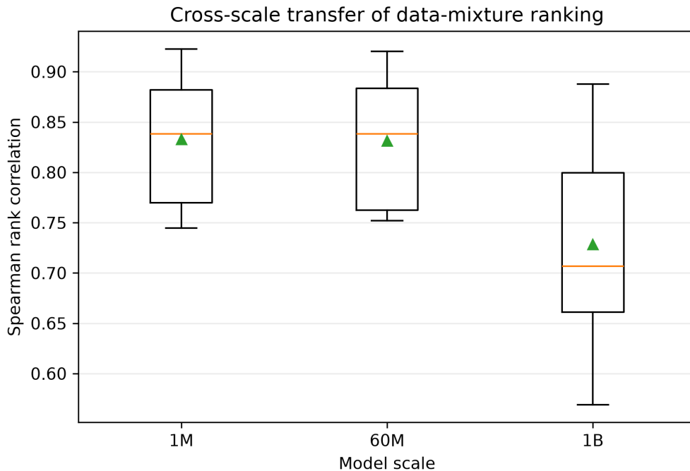
图 3.3 冻结的 1M Ridge 代理在三个真实检验组上的逐目标域排序表现。1B 使用不同的配方集合，因此其变化不能解释为纯参数规模效应。
