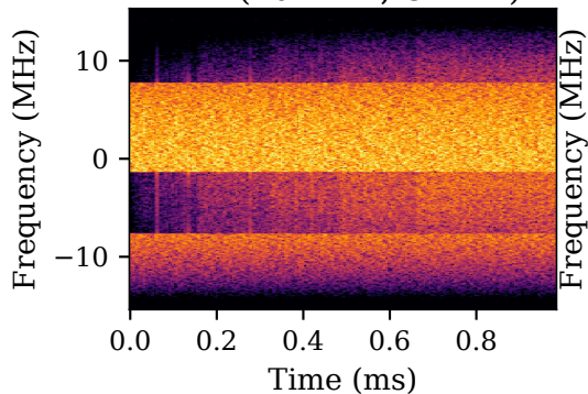
LTE (10 MHz, OFDM)
