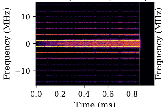
GSM (200 kHz, GMSK)
