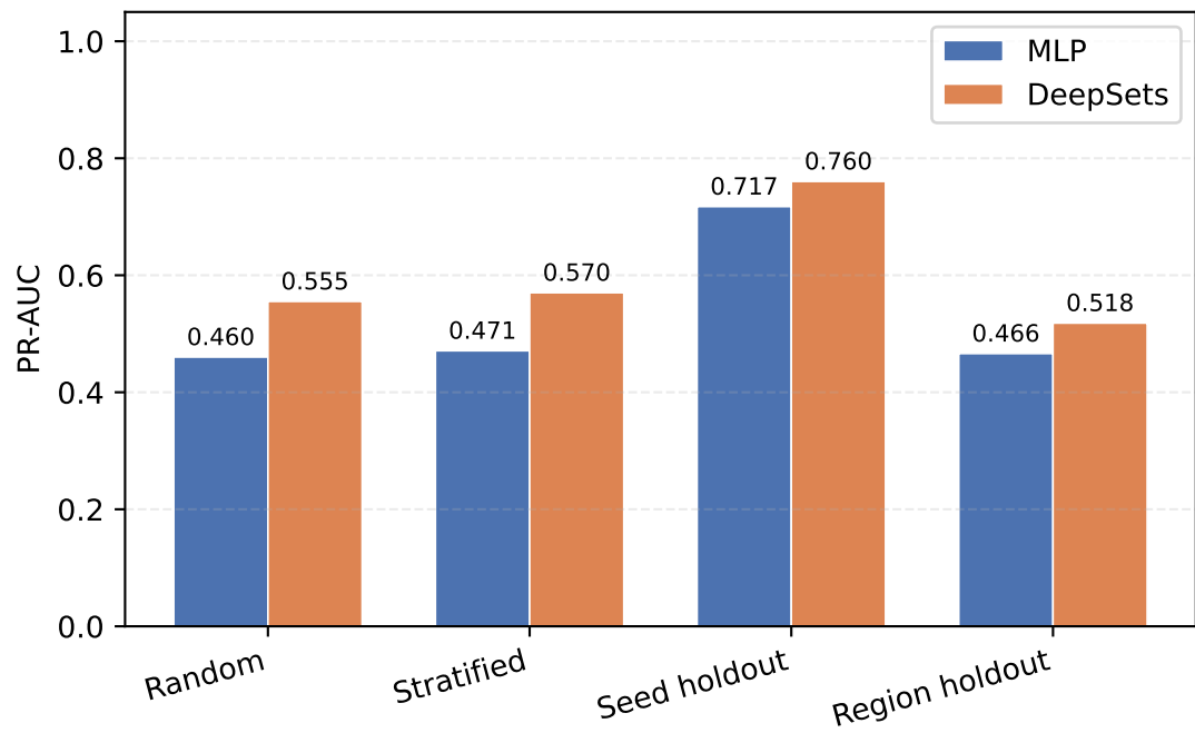
(b) PR-AUC
