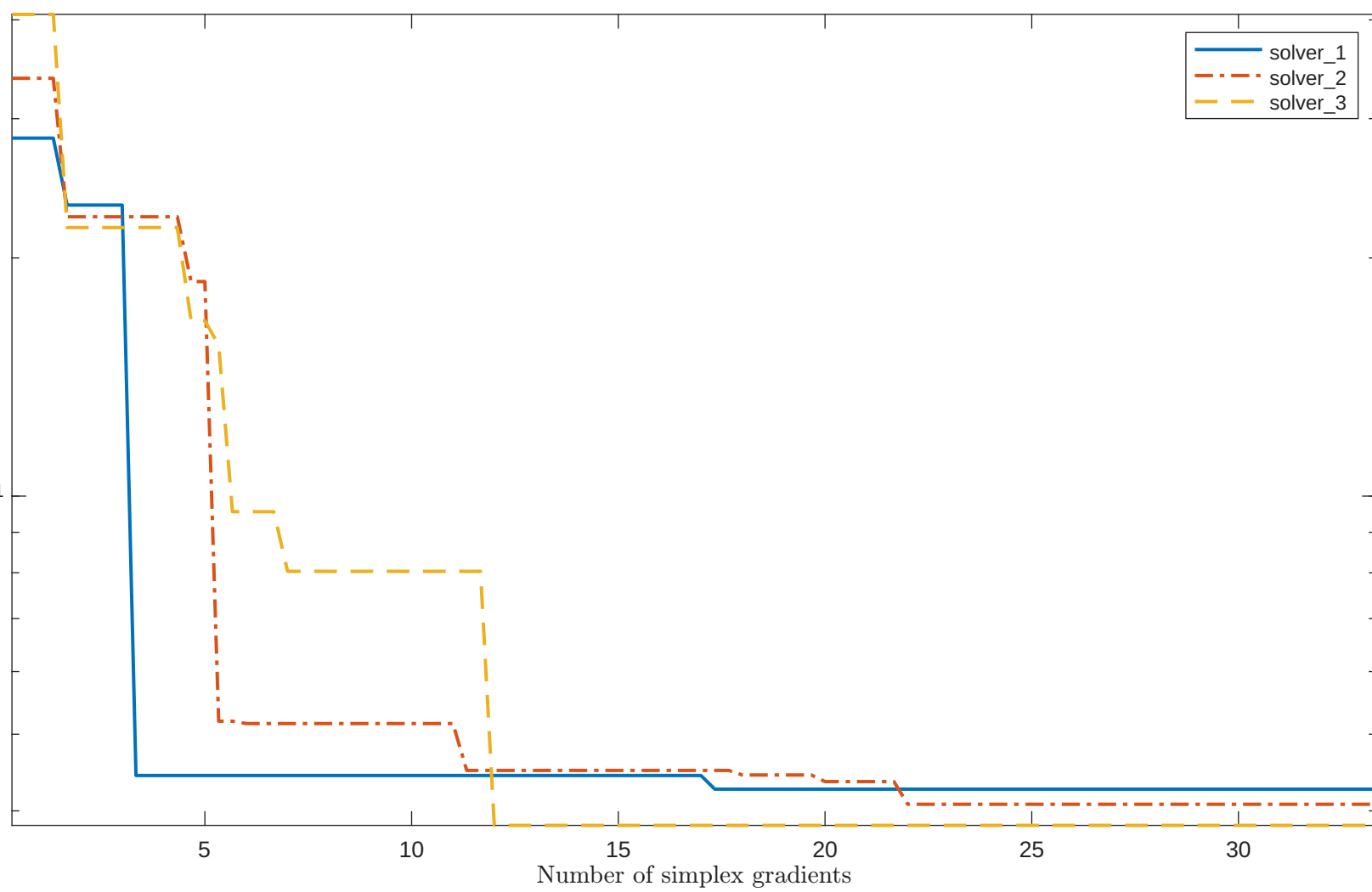
Cummin of function values
