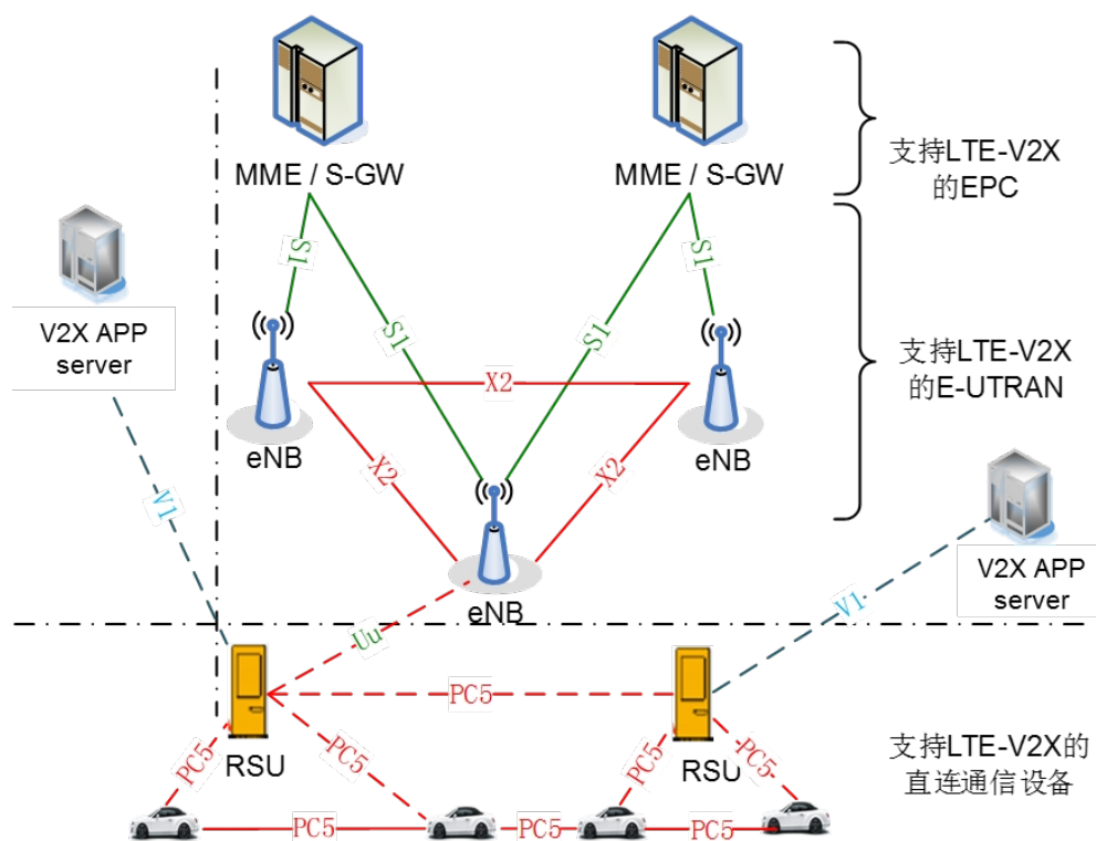
图1 路侧设备在LTE-V2X系统逻辑结构中的位置
