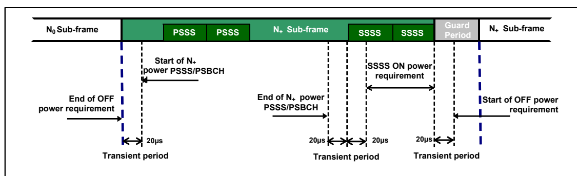
图4 V2X 业务普通 CP 传送 PSSS/SSSS/PSBCH 时间模板
