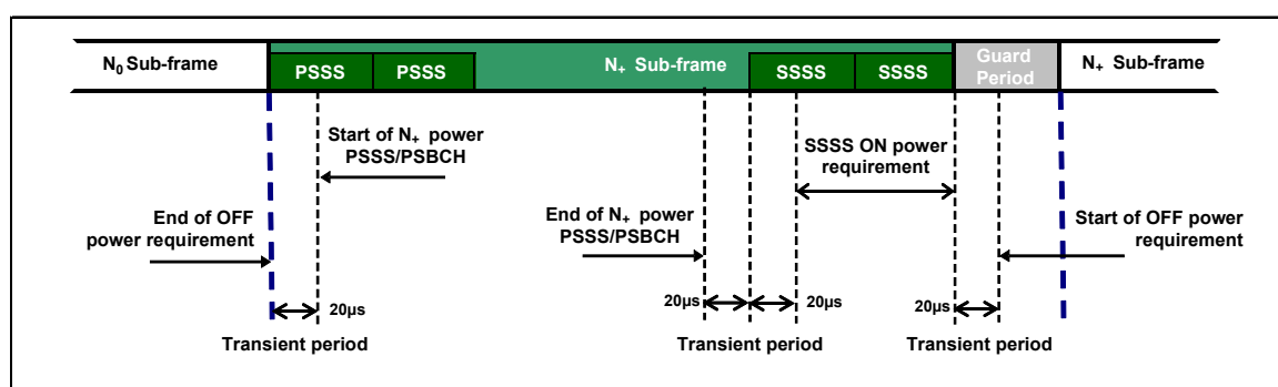
图5 V2X 业务扩展 CP 传送 PSSS/SSSS/PSBCH 时间模板
