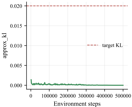
Approximate KL
