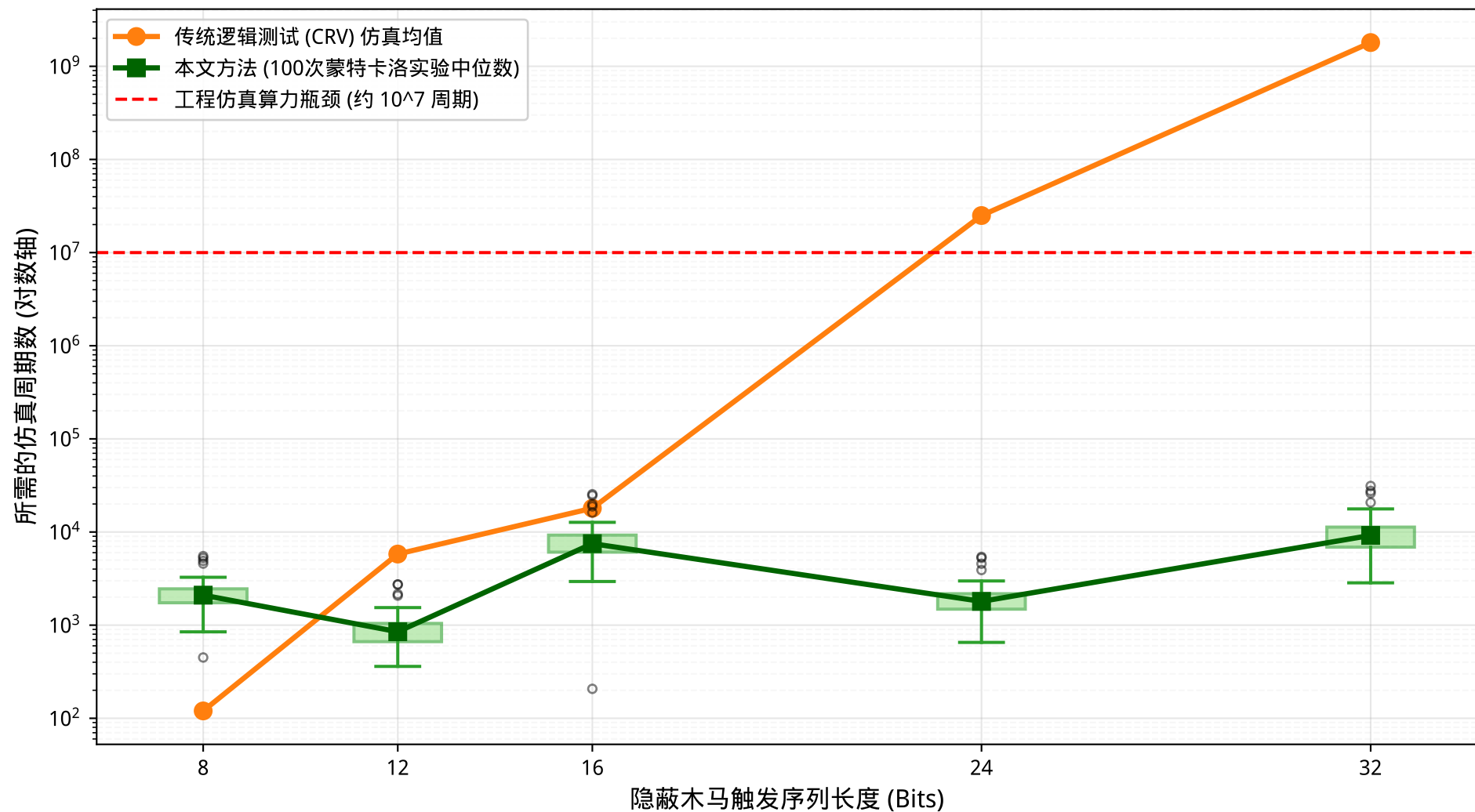
不同激励机制下的隐蔽木马触发开销分布对比
