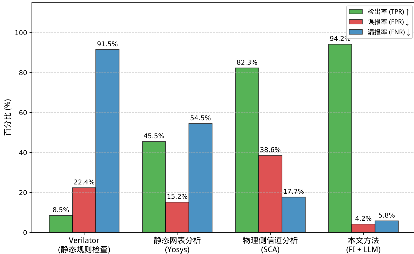
高隐蔽控制路径木马检测性能评估
