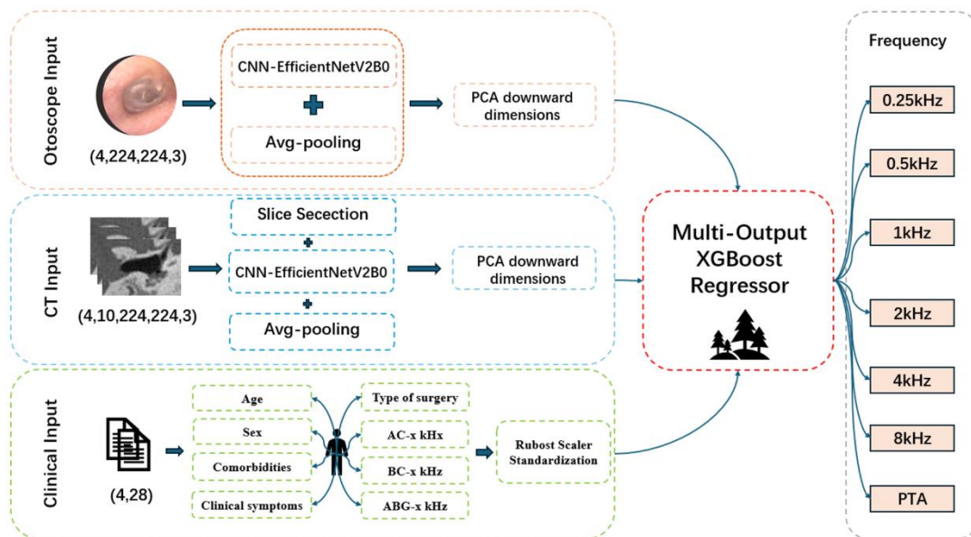
图 1 模型架构图
