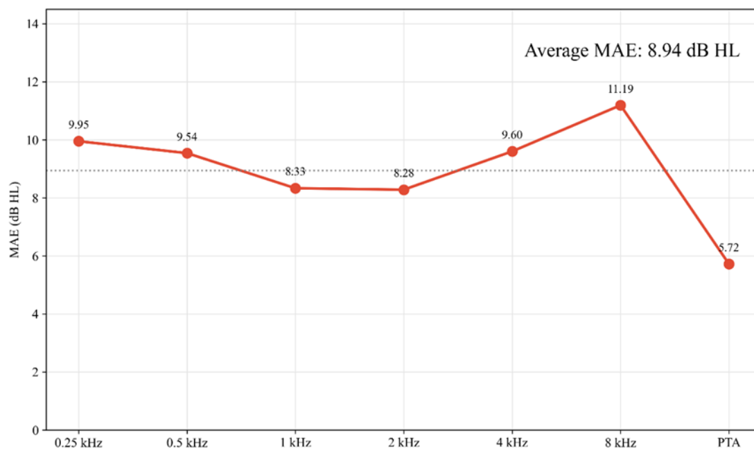
图 2 MAE 折线图
